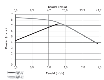
Curva del circulator incluido en la Unidad Interior. Presión disponible a la salida de la bomba de calor
