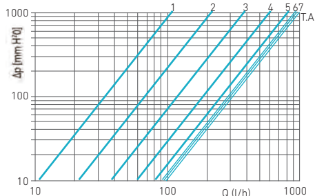
Pérdida de carga del detentor según número de vueltas
