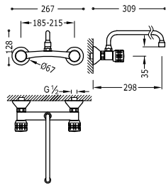
Grifo bimando mural para cocina Con caño superior. Excentricidad especial. Distancia a pared: 298 mm.
