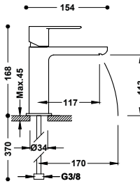
Grifo monomando para lavabo Caño cerrado con salida del agua en cascada. Latiguillos de alimentación flexibles G3/8. Se incluyen 2 llaves de regulación con filtro (ref: 9134525).
