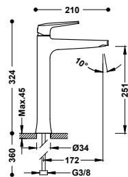
Grifo monomando XXL para lavabo Latiguillos de alimentación flexibles G3/8.
