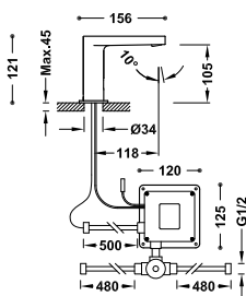
Grifo electrónico con sistema premezclador para lavabo Accionado mediante sensor de infrarrojos. Incluye una válvula mezcladora de 2 aguas con tubos flexibles (ref.: 19250730).
