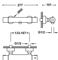
Grifo termostático mural para ducha Ducha de mano anticálcarea: Ø 100 mm. Soporte orientable para ducha de mano. Flexo metálico.
