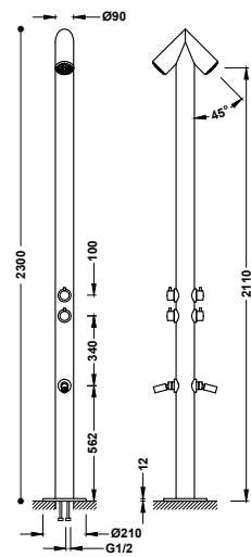
Columna con doble ducha para jardín o piscina de acero inoxidable 316
