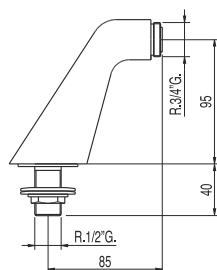
Tomas de agua acodadas de instalación a borde bañera para grifo de bañera 2 unidades con silenciador.
