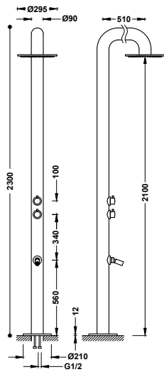
Columna de ducha para jardín o piscina de acero inoxidable 316
