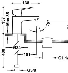
Grifo monomando para lavabo con válvula desagüe Click-Clack Latiguillos de alimentación flexibles G3/8.
